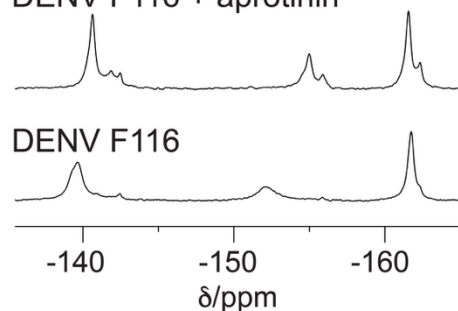
DENV F116 + aprotinin
