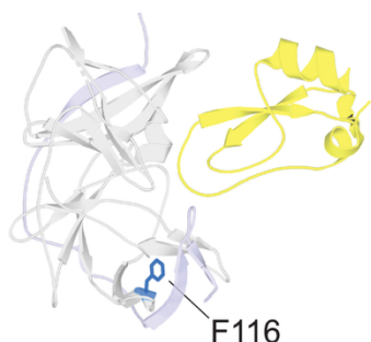
WNV NS2B-NS3 protease
